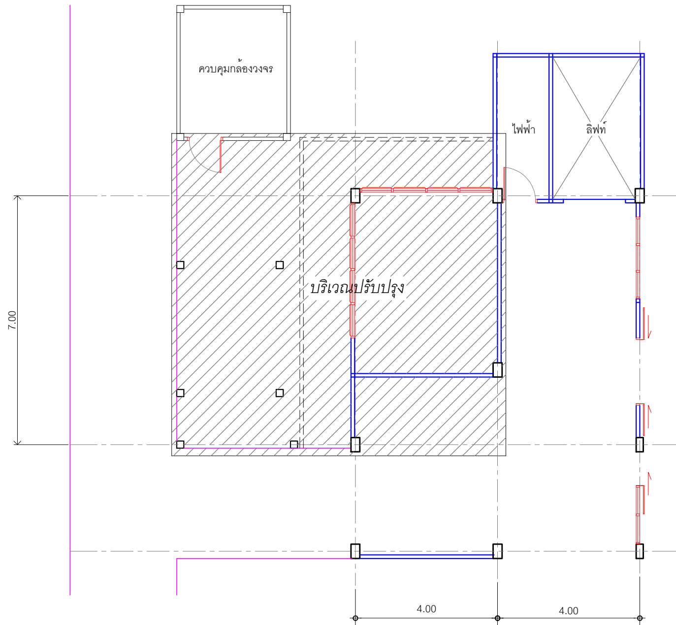
ผังบริเวณในโครงการปรับปรุง ( ตึก 4 ชั้น 1 )
